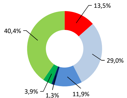
Deutscher Energiemix**
