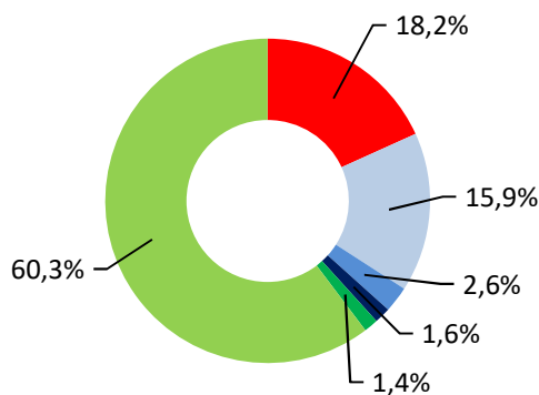
Verbleibender Energiemix*
