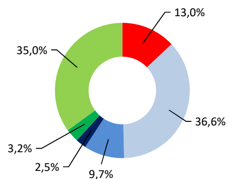
Deutscher Energiemix**
