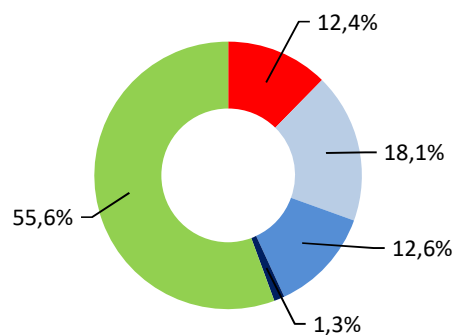
Verbleibender Energiemix*
